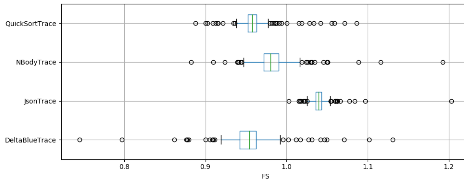
Fig. 4.5: Trazado de código - Factor de sobrecarga
