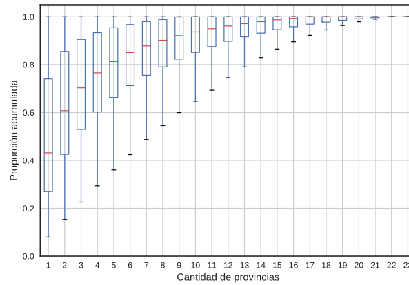
Fig. 3.7: Variación de la proporción de ocurrencias acumulada a partir de la muestra con las primeras 5000 palabras con mayor valor de contrastividad.
