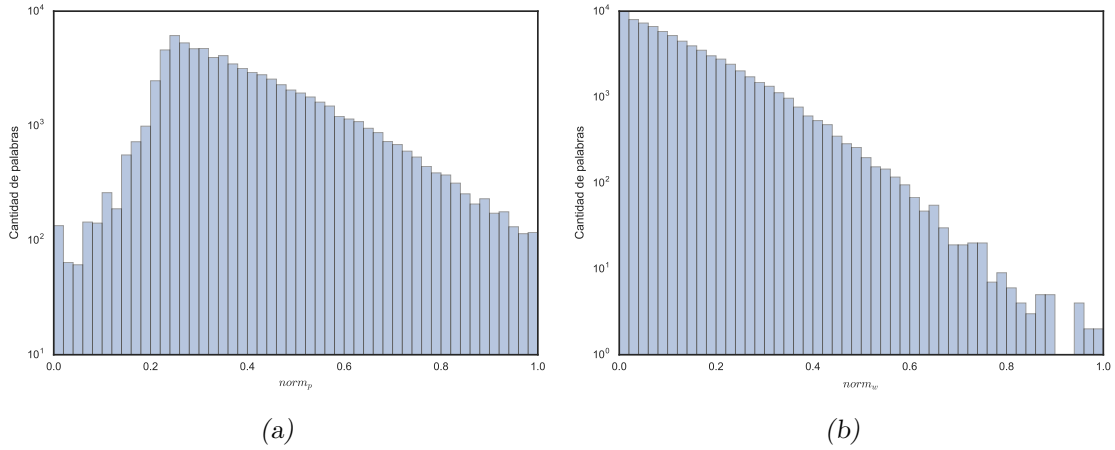
Fig. 3.2: (a) Histograma de la normalización sobre la cantidad de usuarios que utilizan una determinada cantidad de palabras definida como norm_p . (b) Histograma de la normalización de la cantidad de ocurrencias de las palabras definida como norm_w .
