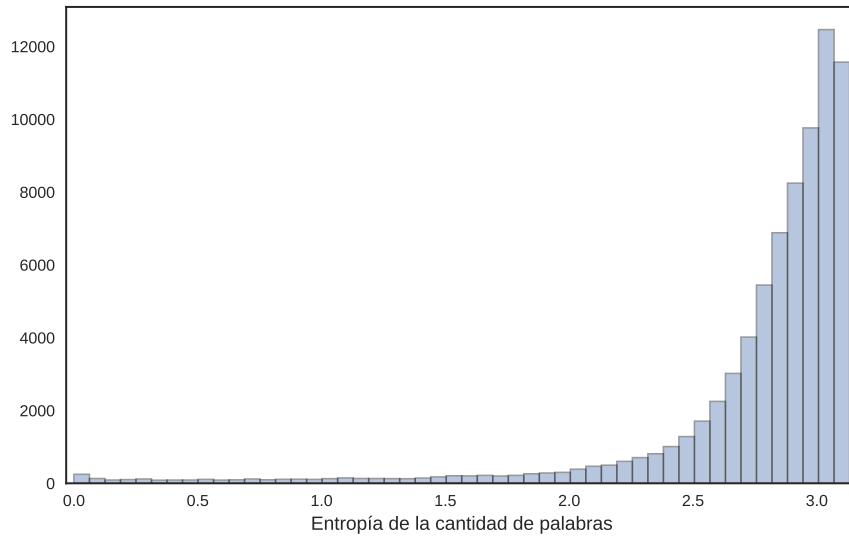
Fig. 3.4: Histograma del valor de la entropía de las palabras ( H_w ).
