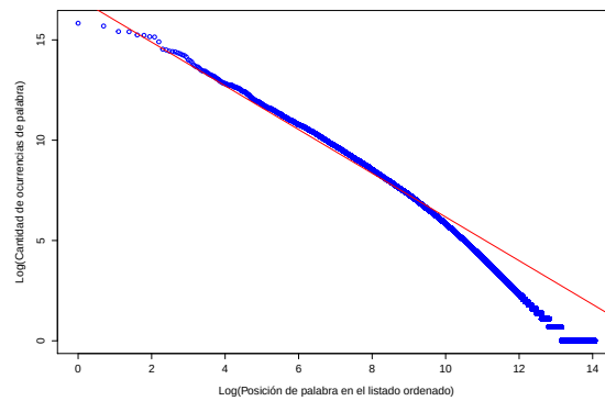
Fig. 3.3: Cantidad de ocurrencias de palabra vs posición en listado ordenado. Se aplicó el logaritmo natural a las cantidades de ocurrencias, como también a los valores de las posiciones para mostrar la proporcionalidad entre f(n) y \frac{1}{n^\alpha} , obteniendo un valor de \alpha = 1,089 .
