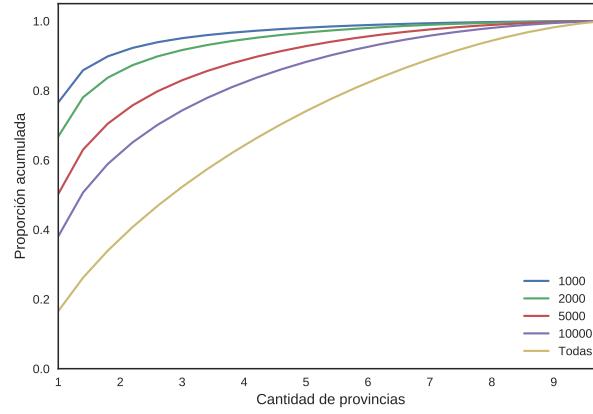
Fig. 3.6: Proporción de ocurrencias acumulada media según la muestra de palabras. El número de la leyenda indica la cantidad de palabras contrastivas elegidas para la muestra respectiva, siempre seleccionando las más contrastivas según la métrica. En cada curva se refleja el promedio de la proporción acumulada de una muestra variando la cantidad de provincias que forman las regiones maximales.
