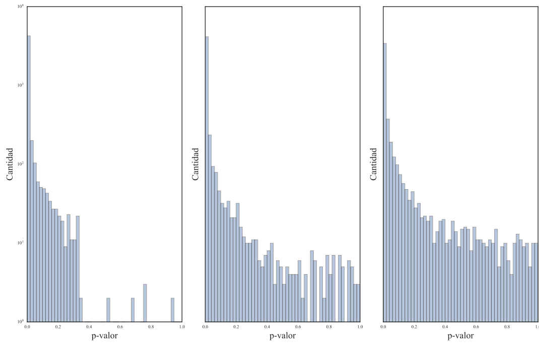
Fig. 4.2: Distribución de p-valores (sin corrección de tests múltiples) en los distintos conjuntos de palabras. De izquierda a derecha se muestran los gráficos dependiendo de los índices de las palabras en el listado ordenado por la métrica del valor de la información: [0,5000] , [20000,25000] , [50000,55000]
