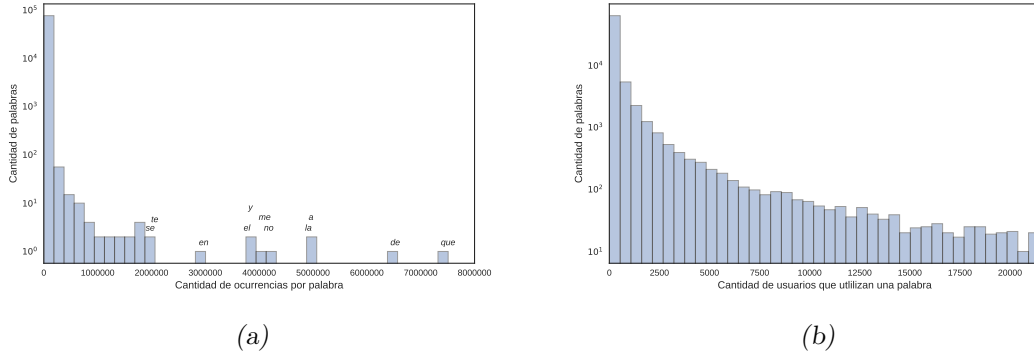
Fig. 3.1: (a) Histograma de la cantidad de ocurrencias de las palabras. (b) Histograma de la cantidad de usuarios que utilizan una determinada cantidad de palabras.
