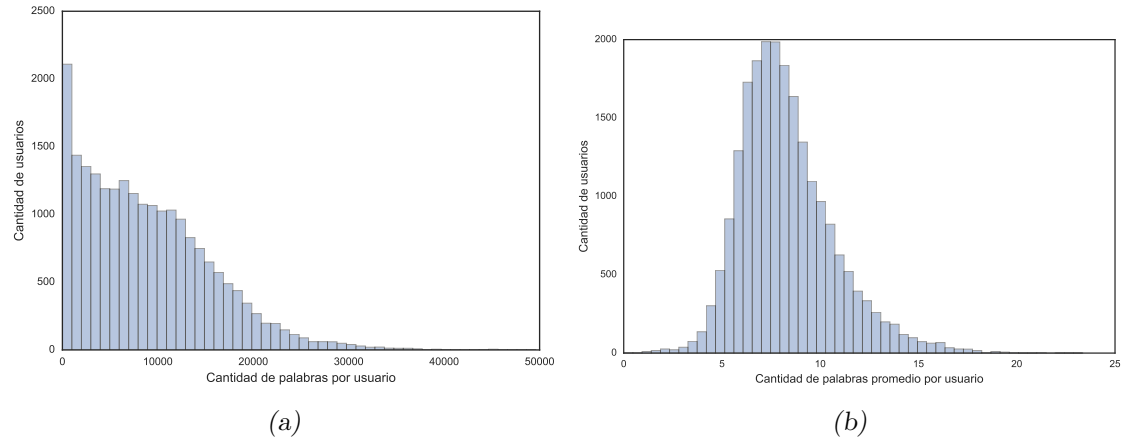
Fig. 2.2: Histogramas: (a) Cantidad de palabras totales por usuario. (b) Cantidad de palabras en promedio por tuit, para todos los usuarios.
