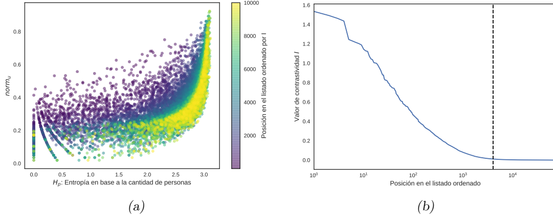
Fig. 3.5: (a) Gráfico de dispersión que muestra la posición en el listado ordenado según el valor de contrastividad reflejado por la escala cromática. A su vez se muestra para cada palabra el valor de la entropía de las personas ( H_p ) y la cantidad normalizada de personas que utiliza dicho término ( norm_p ). (b) Valor de contrastividad según la posición de la palabra en el listado de palabras. El gráfico se realizó sobre el conjunto de palabras cuya cantidad de ocurrencias era mayor a 40 y la cantidad de usuarios que utilizaron cada término era mayor a 5. Desde la palabra cuya posición es 4000, el valor I se estabiliza alrededor de 0.
