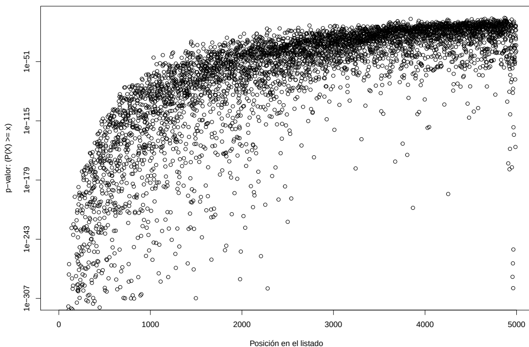
Fig. 4.1: Gráfico de dispersión de los p-valores del test hipergeométrico sobre las primeras 5000 palabras del listado ordenado según la métrica del valor de la información.
