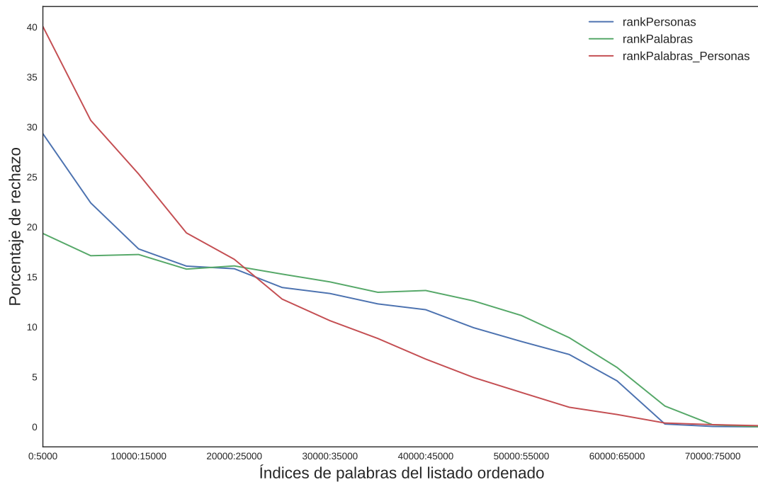
Fig. 4.3: La tasa de rechazo de la hipótesis nula en los distintos conjuntos de palabras, los cuales varían según el índice de estas en el listado ordenado según la métrica elegida.
