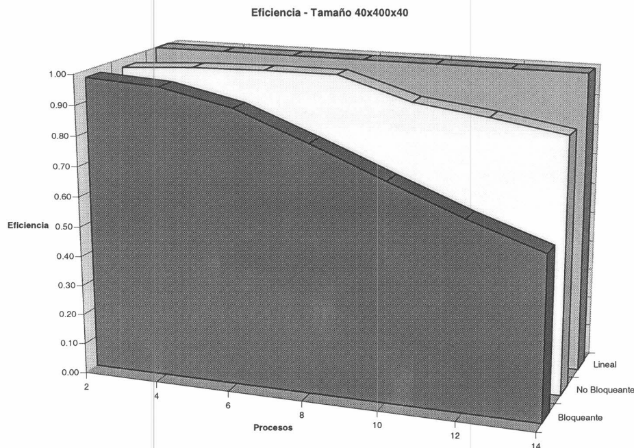
Fig. 5.3.2.2.d – Eficiencia del algoritmo para tamaños de malla 40 \times 400 \times 40
