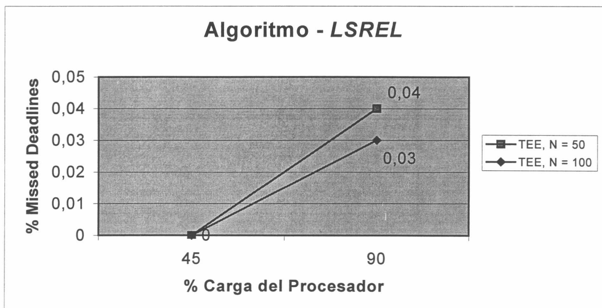
Figura 13 - Resultados con el Algoritmo LSREL para TestExecutionEngine.
