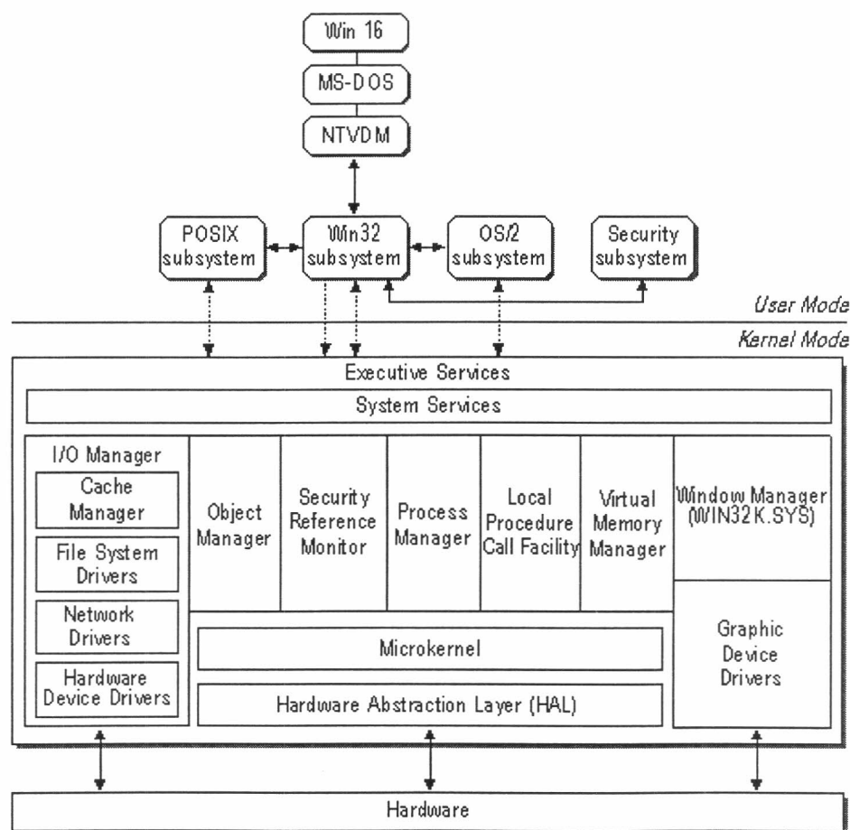
Figura 4 - Arquitectura modular de WindowsNT.
