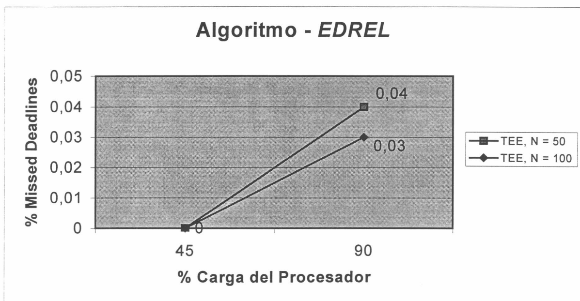
Figura 11 - Resultados con el Algoritmo EDREL para TestExecutionEngine .
