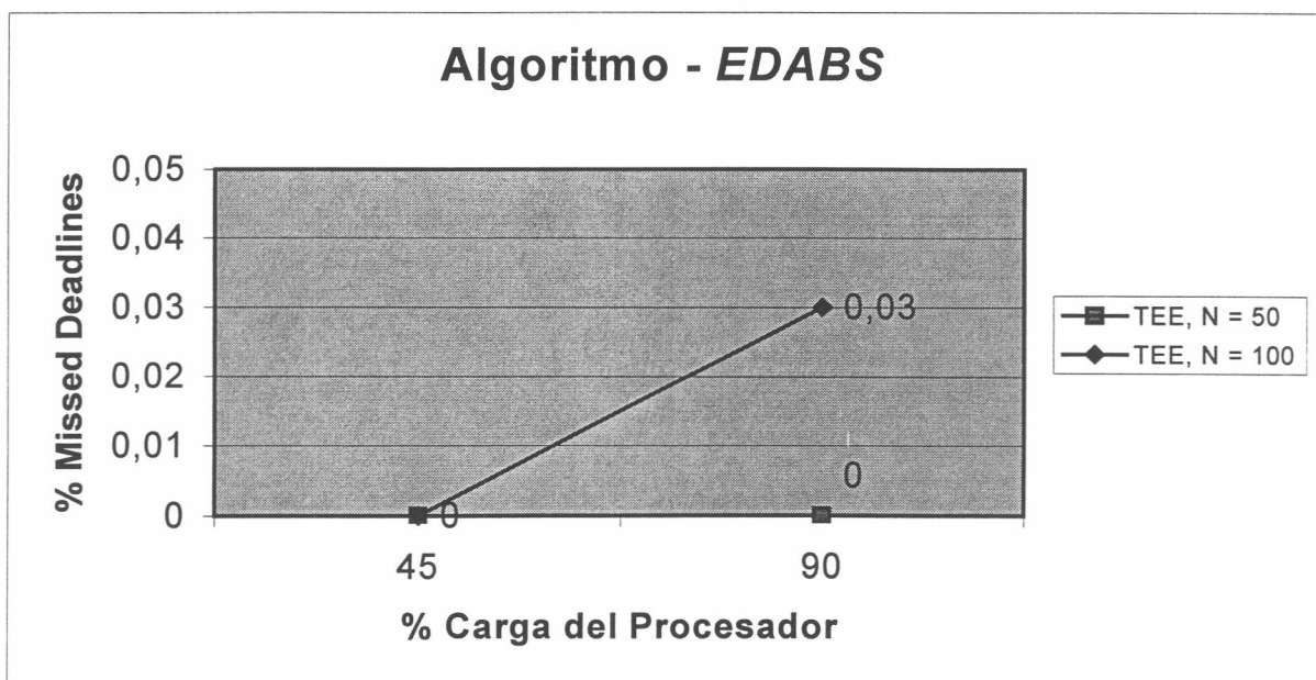
Figura 9 - Resultados con el Algoritmo EDABS para TestExecutionEngine .
