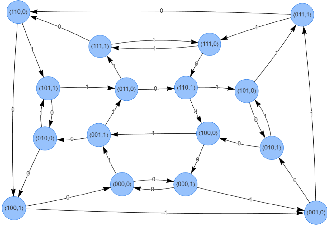
Fig. A.2: Grafo astuto G(3,2)
