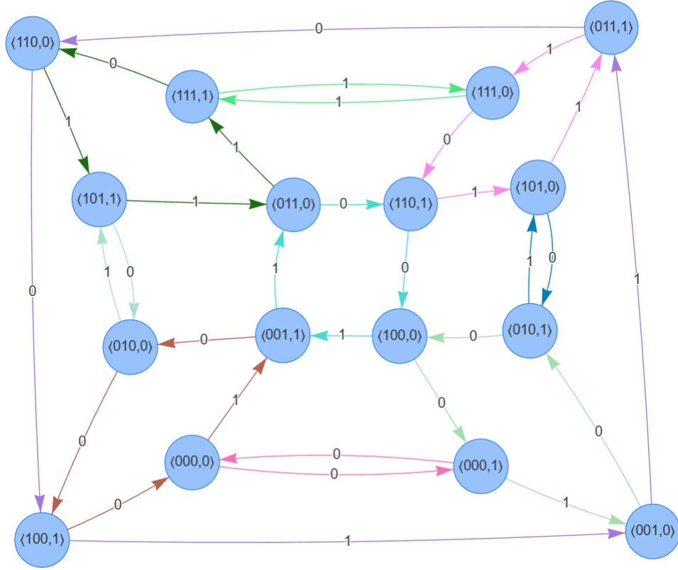
Fig. A.3: Grafo astuto G(3, 2) con los ciclos resaltados por cada par de Lyndon.
