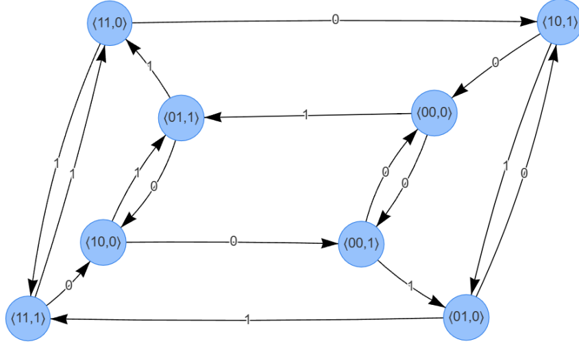
Fig. A.1: Grafo astuto G(2,2)
